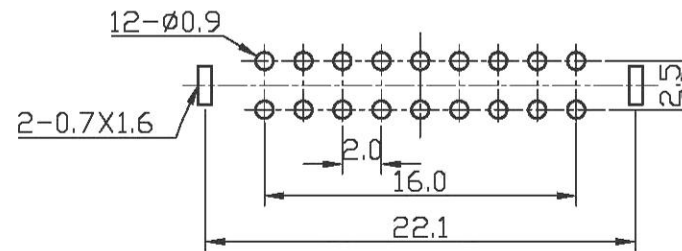
P.C.B. LAYOUT
