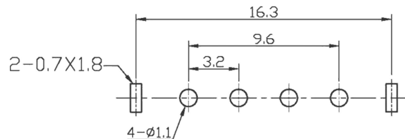
P.B.C. LAYOUT
